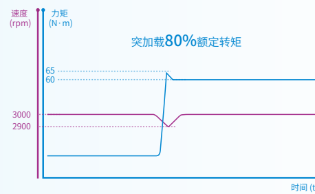
新方案速度&力矩响应曲线
